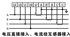
电压直接接入、电流经互感器接入
