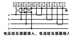
电压经互感器接入、电流经互感器接入
