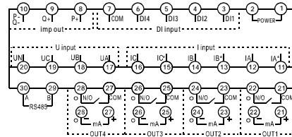
96×96、120×120仪表端子排列及功能定义
